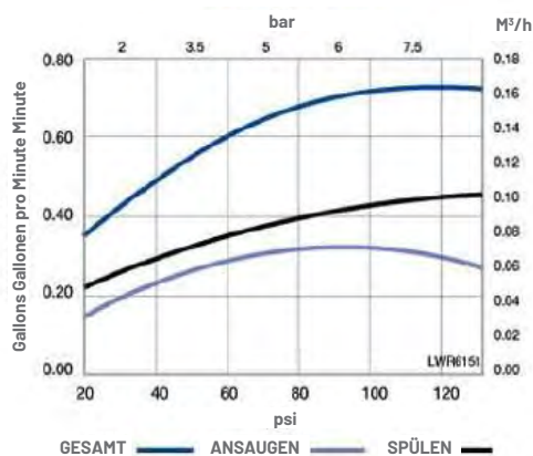
Injektor "J" (hellblau) für 10 Zoll-Tanks
