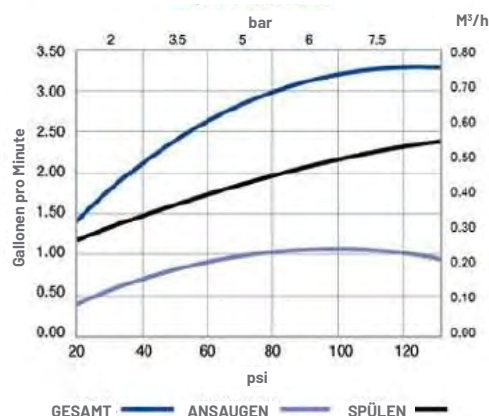
Injektor "R" (dunkel grau) für 21 Zoll-Tanks
