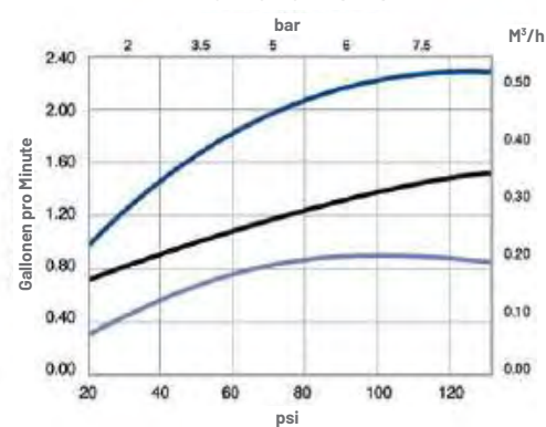
Injektor "R" (dunkel grau) für 21 Zoll-Tanks
