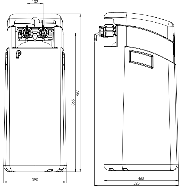
SlimLine CS maxi 1030 28L
